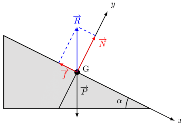
Figure 7.1 – Schéma représentant la situation avec les vecteurs forces appliquées au point G
